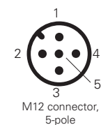
Contact block E1 PNP
